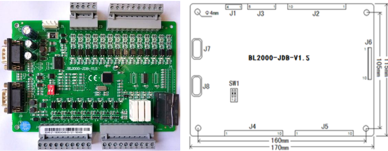
图 3.1 BL2000-JDB-V1. X 轿顶板外形图和安装尺寸
