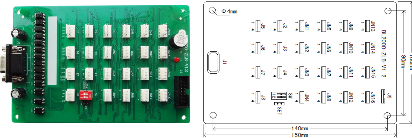
图 3.2 BL2000-ZLB-V1. 2 指令板外形图和安装尺寸
